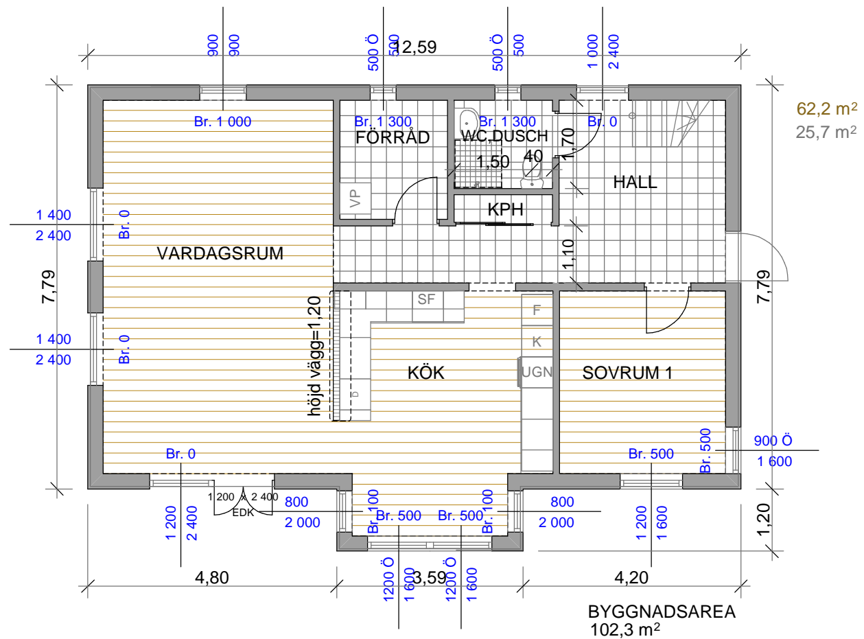
BOTTENVÅNING
